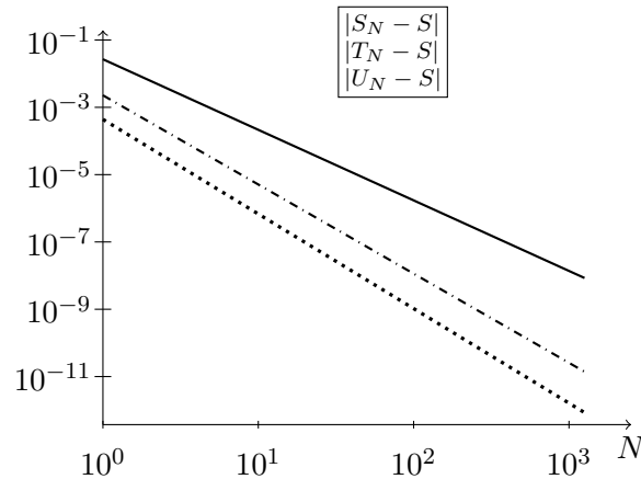
Figure 1 – Évolution des erreurs d'approximation de S par S_N , T_N et U_N .
