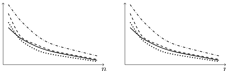
Figure 4 – Évolution des intervalles de confiance pour différentes valeurs de \frac{M}{a} .
