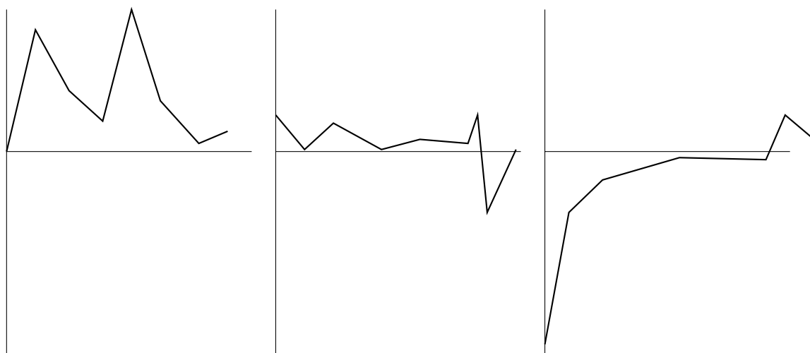
Figure 2 – Trois réalisations de (\bar{X}_1, \dots, \bar{X}_n) .
