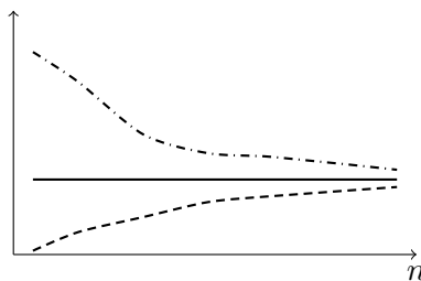
Figure 3 – Évolution des intervalles de confiance pour a = M = 1 .
